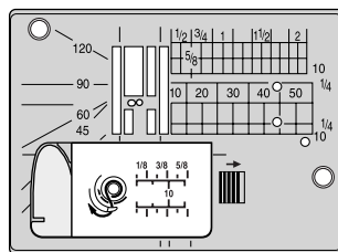
直線ぬい用針板 〈29 ページ参照〉
